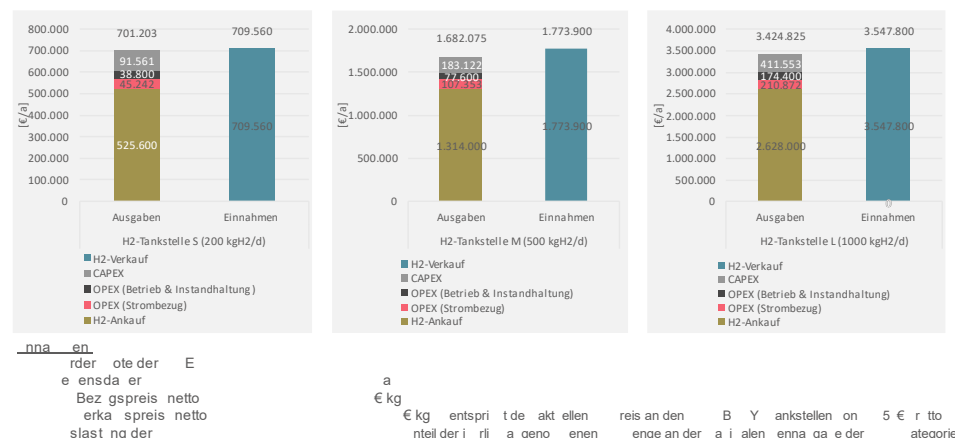
Abbildung 53: Jährliche Ausgaben und Einnahmen der Tankstellengrößen S, M und L; Quelle: Berechnungen BBHC
