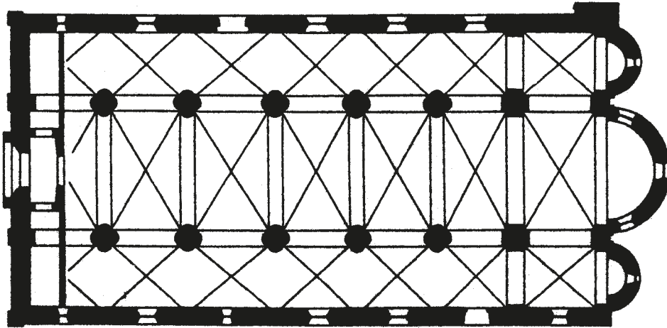
Grundriss der Basilika von Altenstadt
