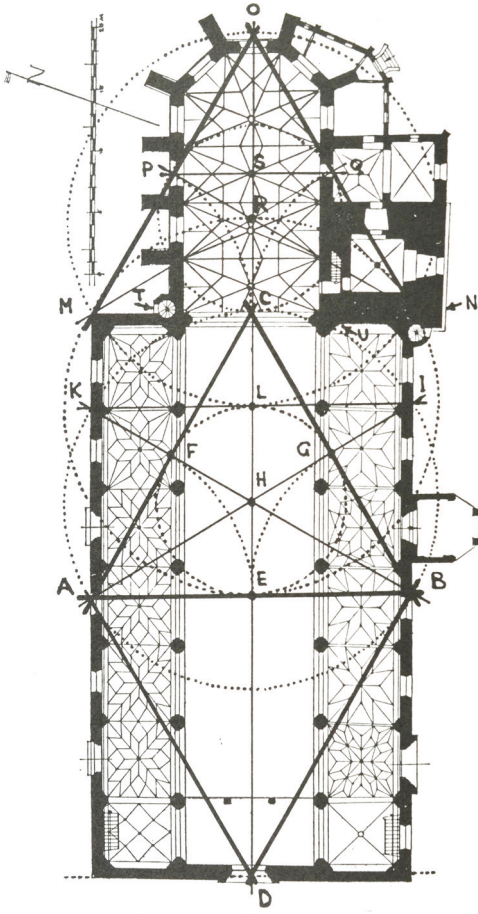
Darstellung der Triangulatur von St. Martin (A. Brenner)
