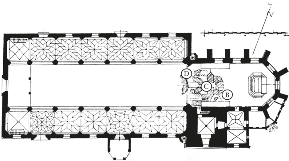
Lageplan der ergrabenen Vorgängerapsiden von St. Martin (Ausgrabungsbericht in: KGBI, Band 9, Seite 60)
