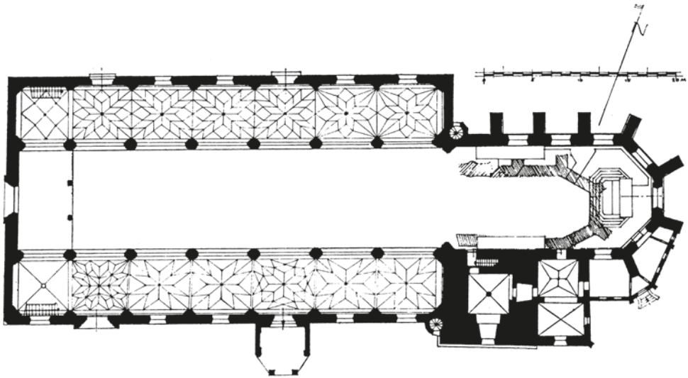
Ergrabener Chor der Vorgängerkirche des 14. Jahrhunderts (Ausgrabungsbericht in: KGBI, Band 9, Seite 60)
